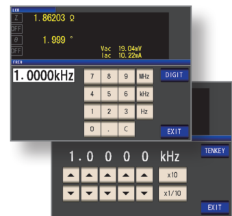
주파수 설정 (10개 버튼 입력과 업 다운 입력)
