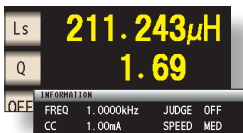
L, Q 표시하면 (1 kHz, CC 1 mA 측정)
