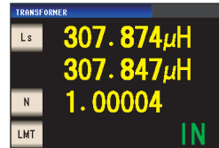
트랜스 측정 모드 권수비 측정 · 판정화면
